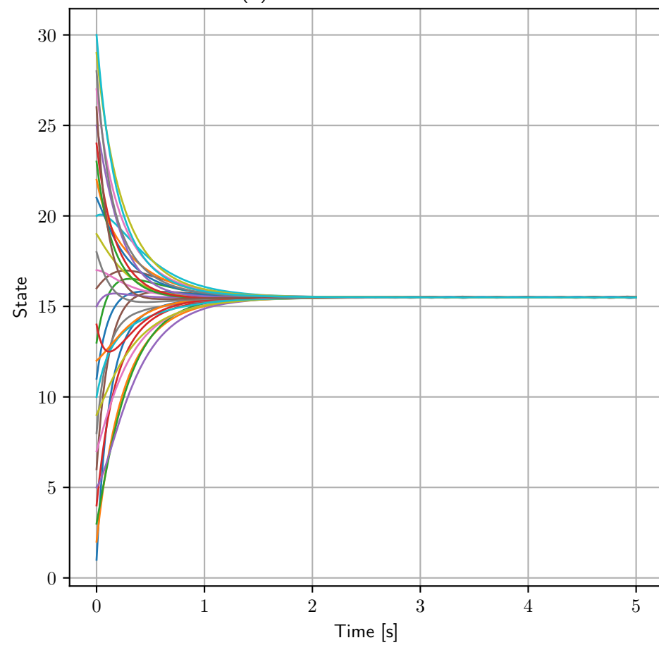
(d) Consensus: Small-world
